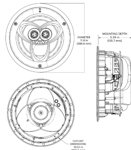
DC-80 MAX SUR
